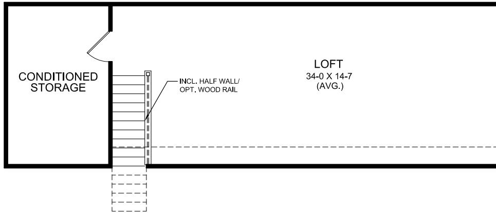
OPTIONAL LOFT DESIGN
